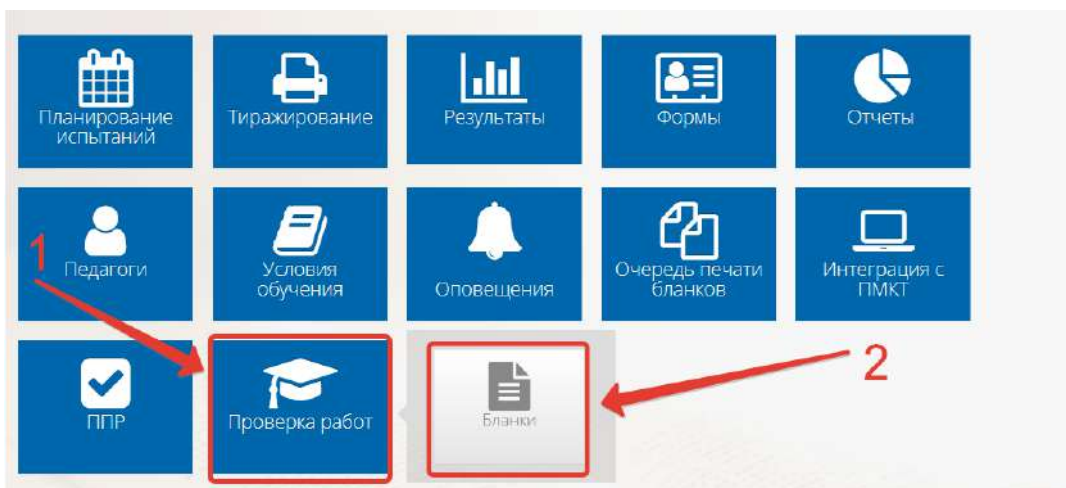
Рисунок 27. Бланки
