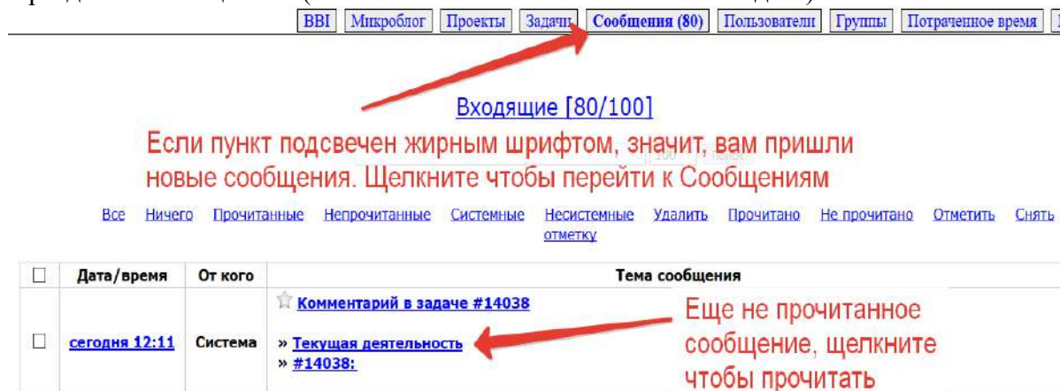
Рисунок 45. Система сообщений
