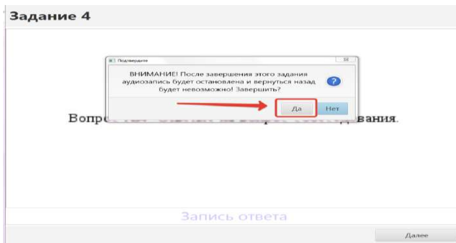
Рисунок 62. Завершение собеседования
