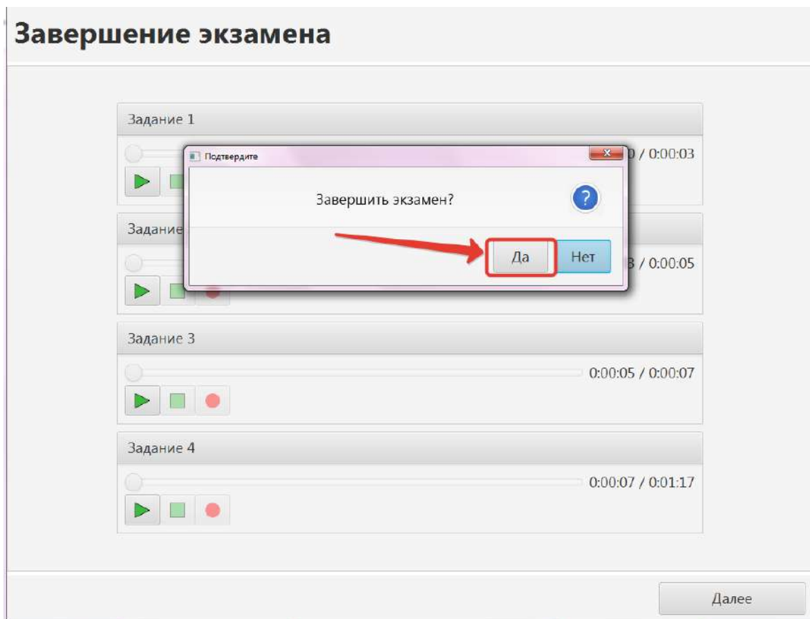
Рисунок 64. Завершение собеседования
