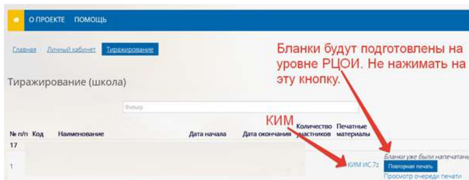
Рисунок 16. Скачивание КИМ
