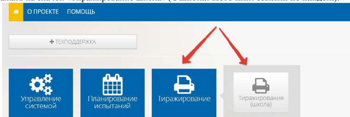
Рисунок 15. Тиражирование (школа)
