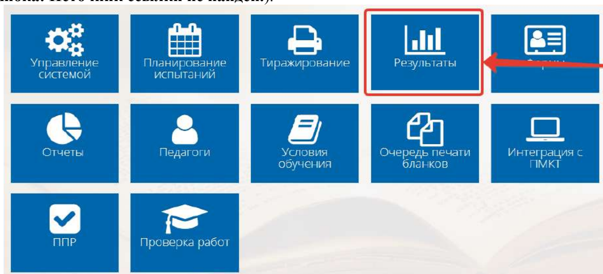
Рисунок 37. Вкладка «Результаты»
