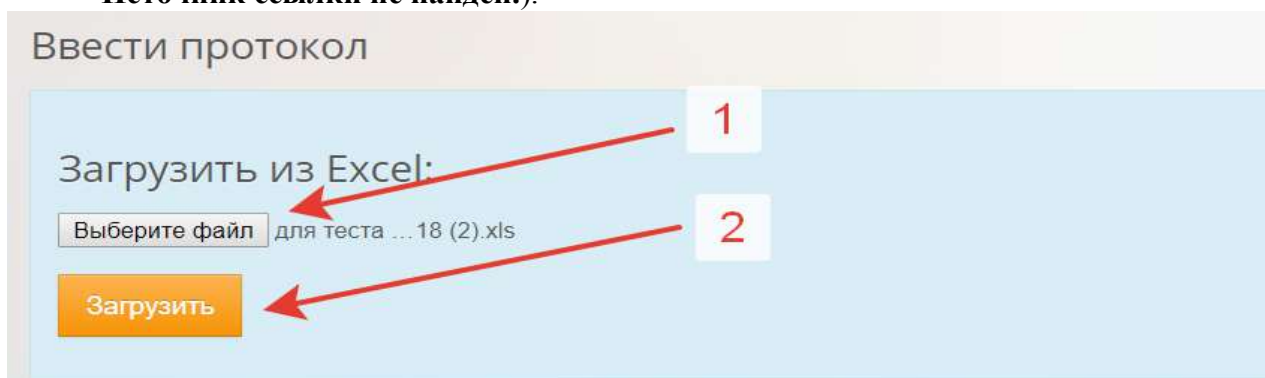
Рисунок 34. Загрузка файла
