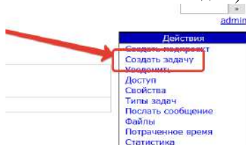
Рисунок 43. Создание задачи
