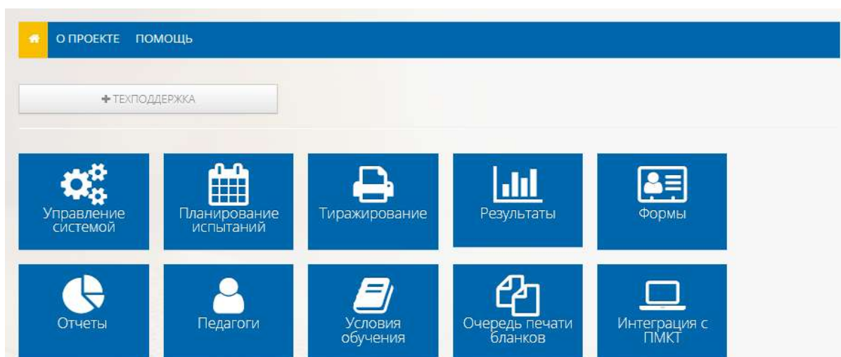
Рисунок 9. Интерфейс системы
