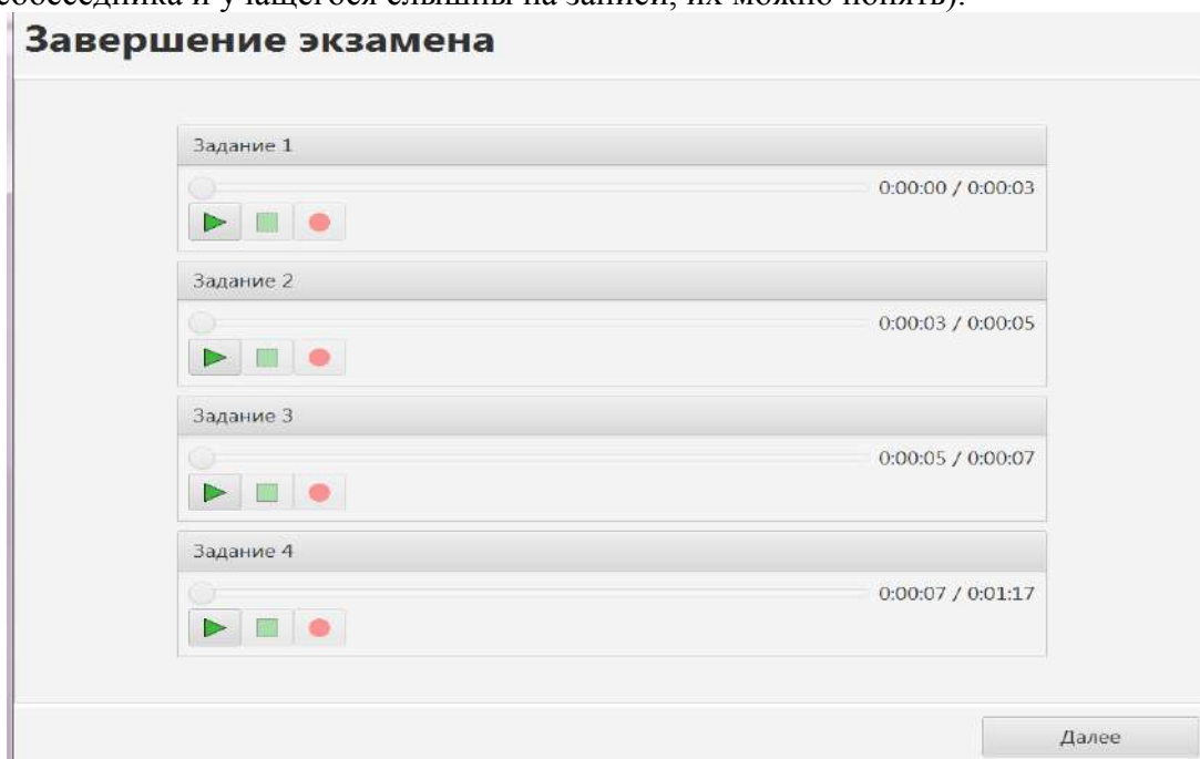
Рисунок 63. Проверка ответов
