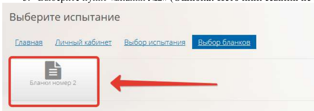
Рисунок 28. Бланки №2
