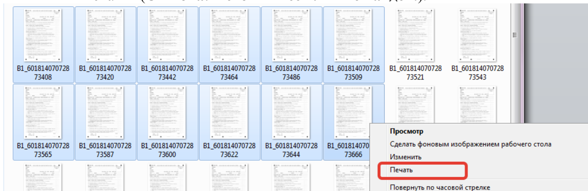
Рисунок 12. Печать
