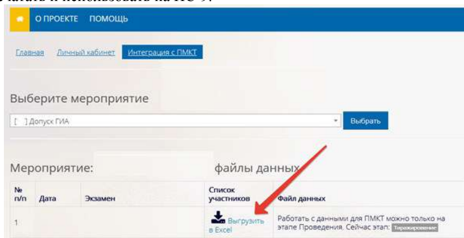
Рисунок 14. Выбор испытания
